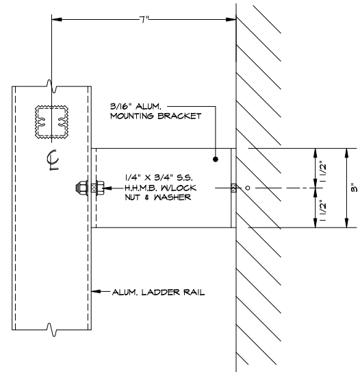
WALL BRACKET SCALE: 3"=1'-0"
