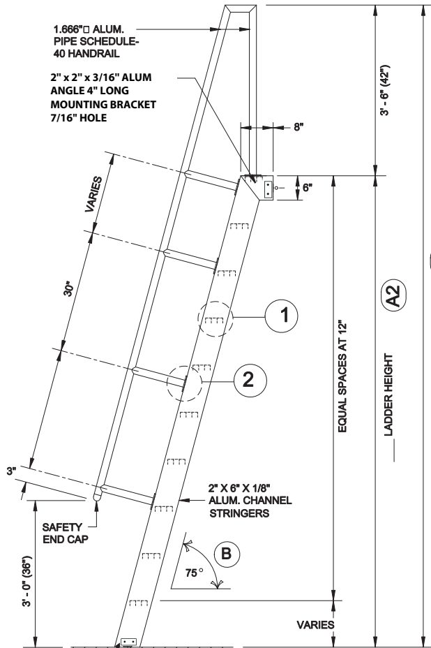
SIDE ELEVATION N.T.S.
