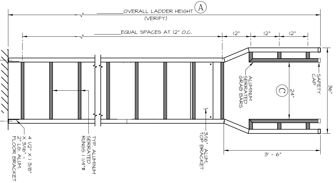
FRONT ELEVATION N.T.S.
