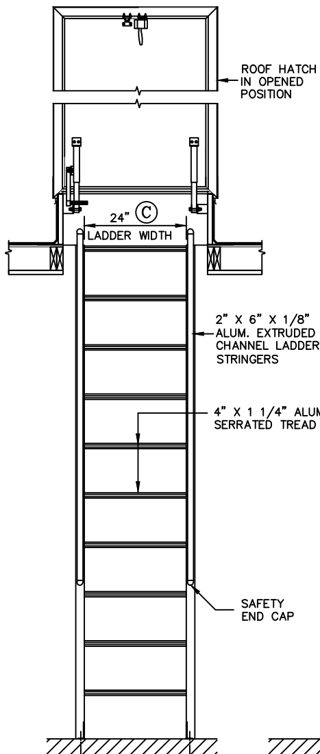
FRONT ELEVATION N.T.S.
